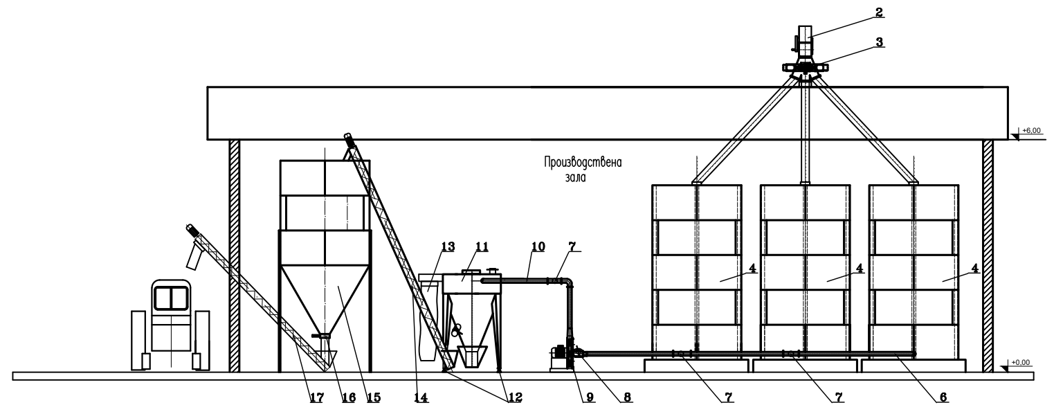
РАЗРЕЗ 1 - 1
